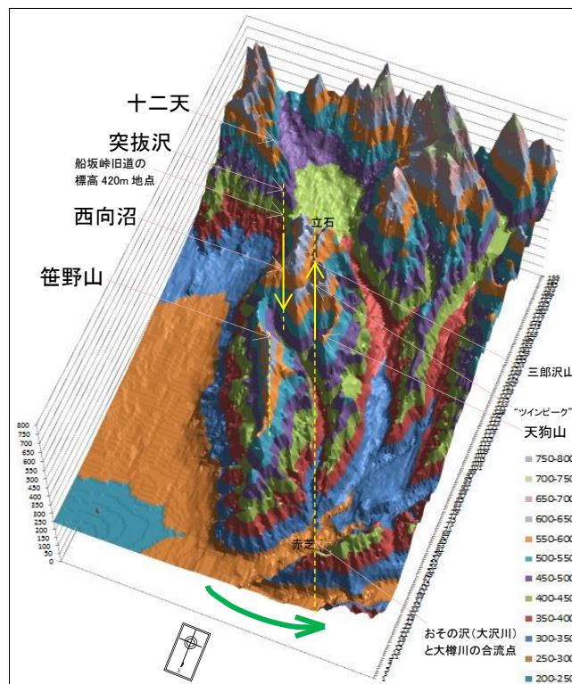
図 1. N22°W の平行線(黄色い矢印は左横ずれ断層, 緑色の矢印は反時計回りの回転. 平 27 情使, 第 322 号).
